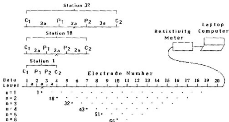
Illustration II.3.1 C - Schéma de construction de la pseudo-section, d'après Loke, 1997.
