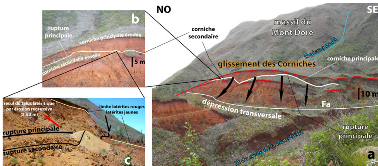
Illustration III.4.2 E - Le glissement des Corniches (Cor) et la faille Fa.
