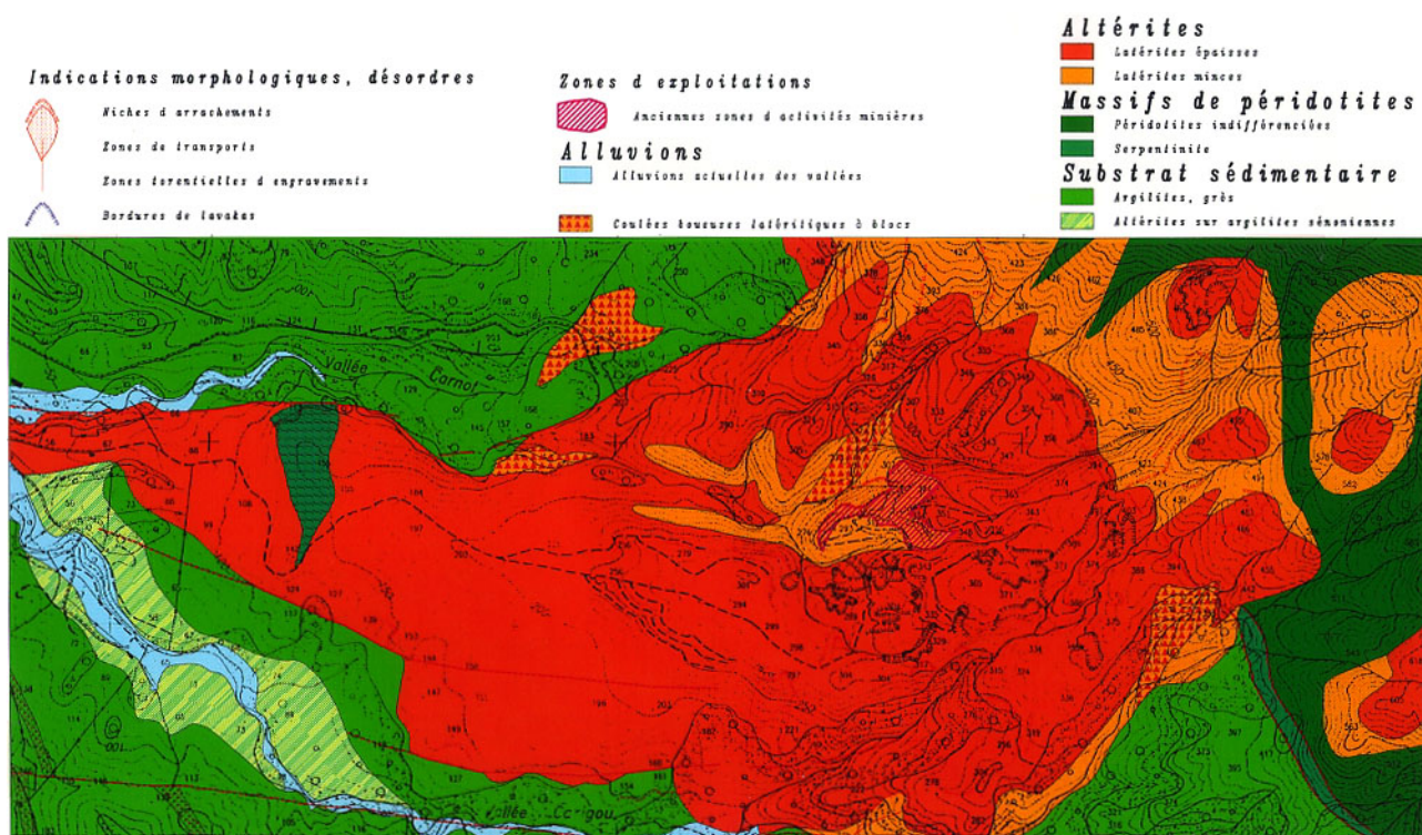
Illustration IV.2.3 C - Carte géologique au 1/10 000 des masses glissées dans la Vallée Carnot, au pied des monts Koghi. Maurizot & Lafoy, 1998b.
