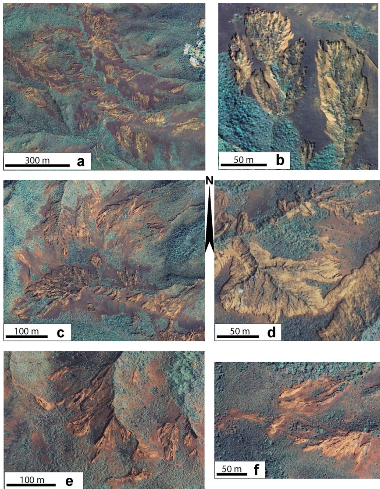
Illustration I.4.1 E: Vues aériennes de lavakas en milieu ultrabasique néocalédonien (images Géorépertoire NC) a, b, c : bassin de la Coulée d : monts Koghi e, f : bassin de la Dumbéa
