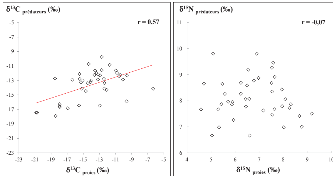
Figure 5.11 : Régressions linéaires entre les signatures isotopiques ( \delta^{13}\text{C} et \delta^{15}\text{N} , ‰) des prédateurs et celles de leurs proies, G. chilospilus , Conger L1 et Conger Ls confondues.
