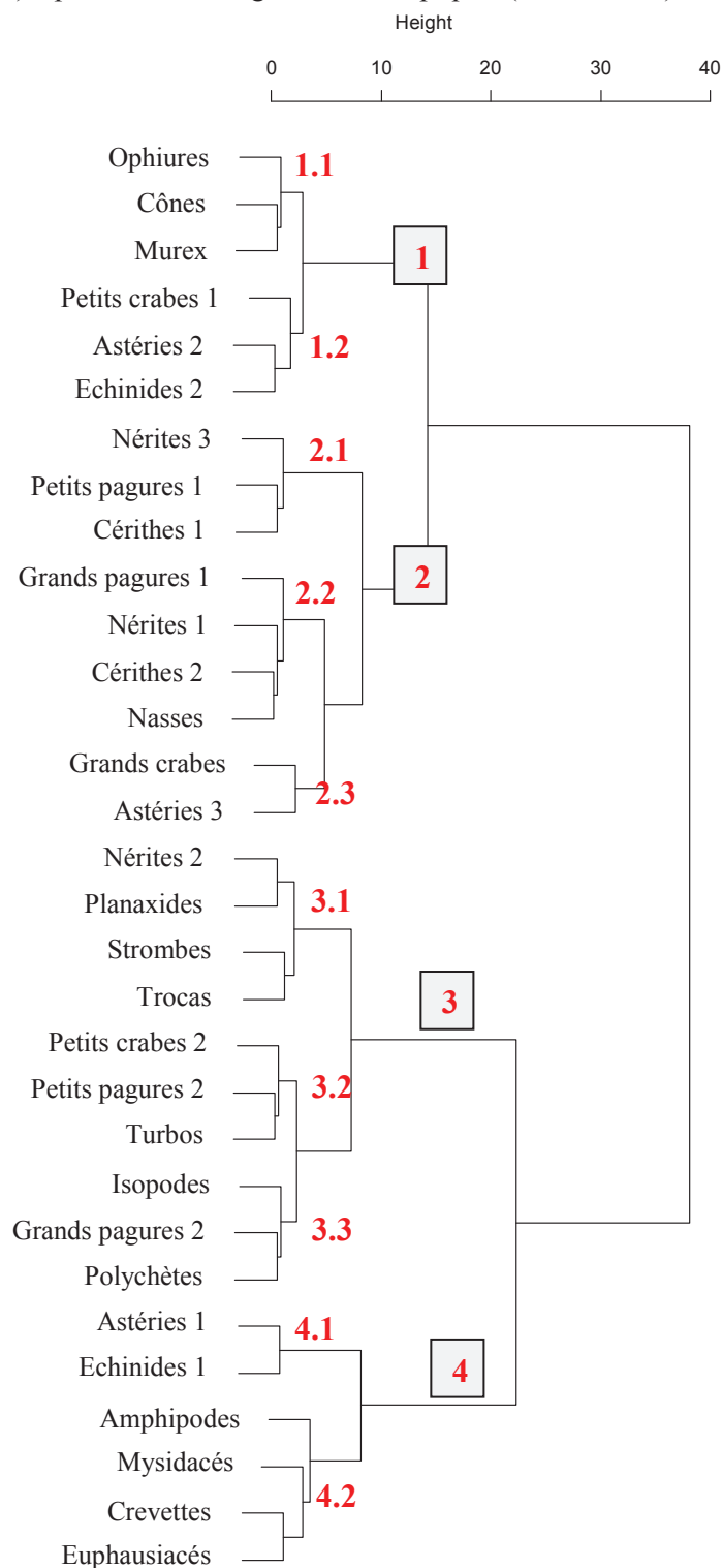
Annexe 4.6 – Dendrogramme des groupes d'invertébrés obtenu par classification hiérarchique ascendante (ACH) à partir de leurs signatures isotopiques ( \delta^{13}\text{C} et \delta^{15}\text{N} ).
