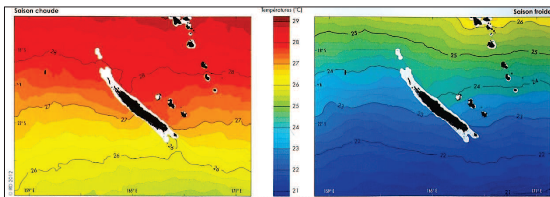
Figure 1.2 : Températures moyennes des eaux de surface autour de la Nouvelle-Calédonie, en été austral (gauche) et en hiver austral (droite) (Données de la NOAA pour la période 1982-2000, IRD 2012).
