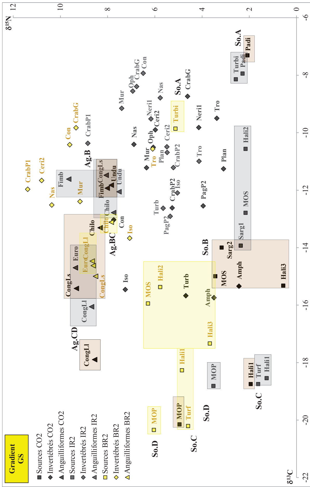
Figure 6.4 : Structure des réseaux trophiques récifo-lagonaires le long du gradient côte-large du Grand Lagon Sud (côte « CO2 », intermédiaire « IR2 », barrière « BR2 »). La variabilité spatiale des signatures isotopiques des sources (So) et des poissons anguilliformes (Ag) impliqués dans les voies de transfert A à D est mise en évidence (rectangles) par un code couleur correspondant aux différents sites ( Codification des organismes en Annexe A ).
