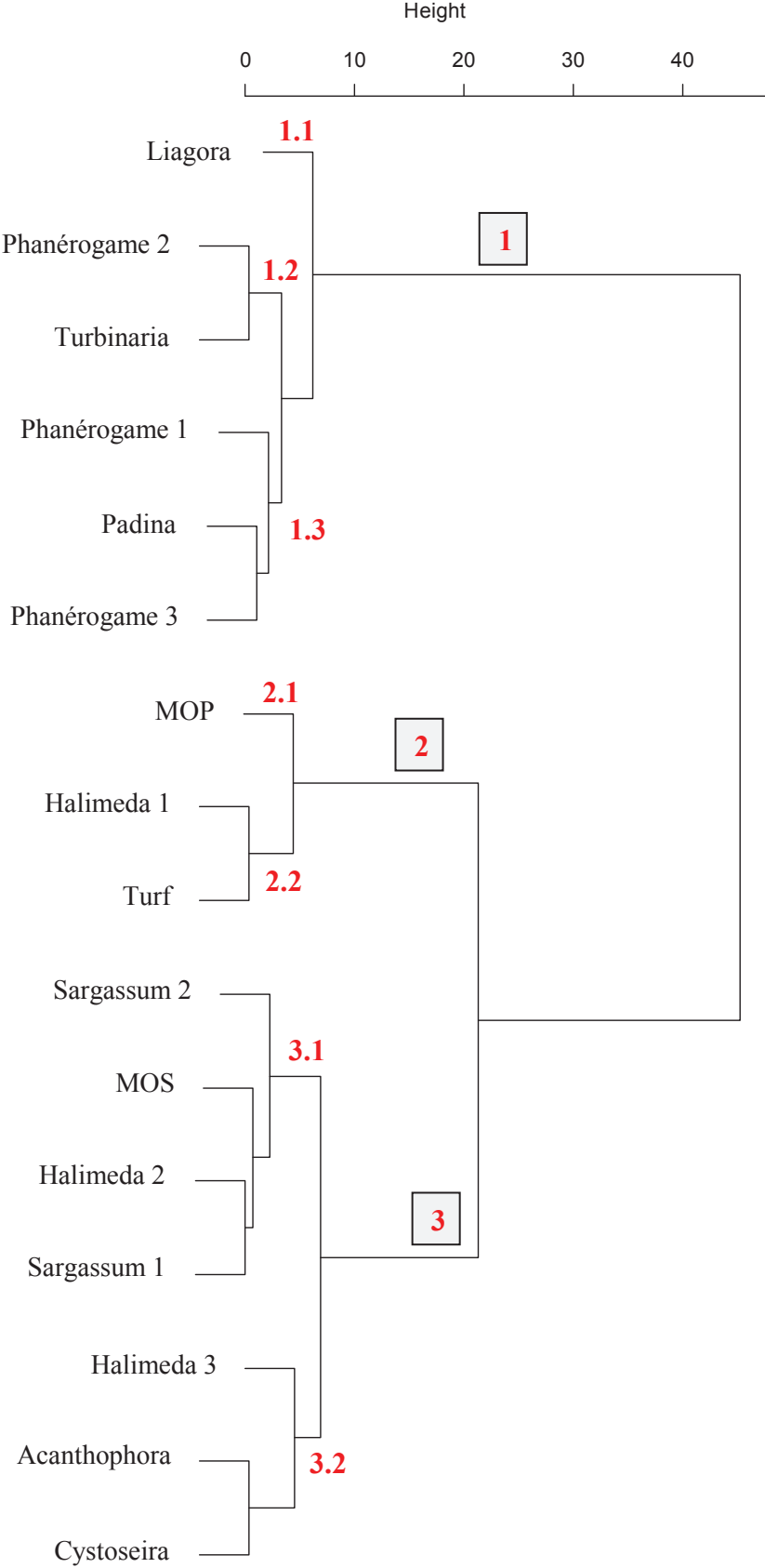
Annexe 3.5 - Dendrogramme des sources potentielles de MO des écosystèmes récifo-lagonaires (réservoirs et producteurs primaires) obtenu par classification hiérarchique ascendante (ACH) à partir de leurs signatures isotopiques ( \delta^{13}\text{C} et \delta^{15}\text{N} ).
