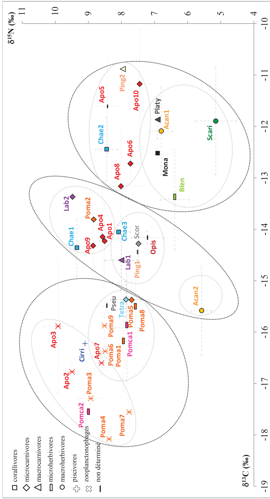
Figure 4.6 : Représentation graphique des signatures isotopiques en carbone ( \delta^{13}\text{C} ) et en azote ( \delta^{15}\text{N} ) des poissons : Acanthuridae (jaune), Apogonidae (rouge), Bleenniidae (vert clair), Chaetodontidae (bleu foncé), Cirrhitidae (bleu clair), Labridae (violet), Monacanthidae (noir), Opistognathidae (rouge foncé), Pinguipedidae (beige), Platycephalidae (marron), Pomacanthidae (rose), Pocamantidae (orange), Pseudo (vert kaki), Scaridae (vert foncé), Scorpaenidae (gris), Tetraodontidae (bleu ciel). Les sept groupes trophiques (corallivores, microcarnivores, macrocarnivores, microherbivores, macroherbivores, piscivores, zooplanctonophages) sont symbolisés sur le graphique. Les écarts-types sont représentés par les barres d'erreurs en pointillés. Les cercles pointillés symbolisent les groupes et sous-groupes de poissons obtenus par les analyses CAH.
