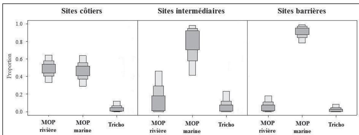
Figure 3.3 : Importance relative de la MOP de rivière, de la MOP marine lagonaire et des blooms de Trichodesmium spp. dans la composition isotopique de la MOP aux sites côtiers, intermédiaires et barrières du lagon. Les boîtes représentent 50%, 75% et 95% (du gris sombre au gris clair) des intervalles de crédibilité Bayésien.
