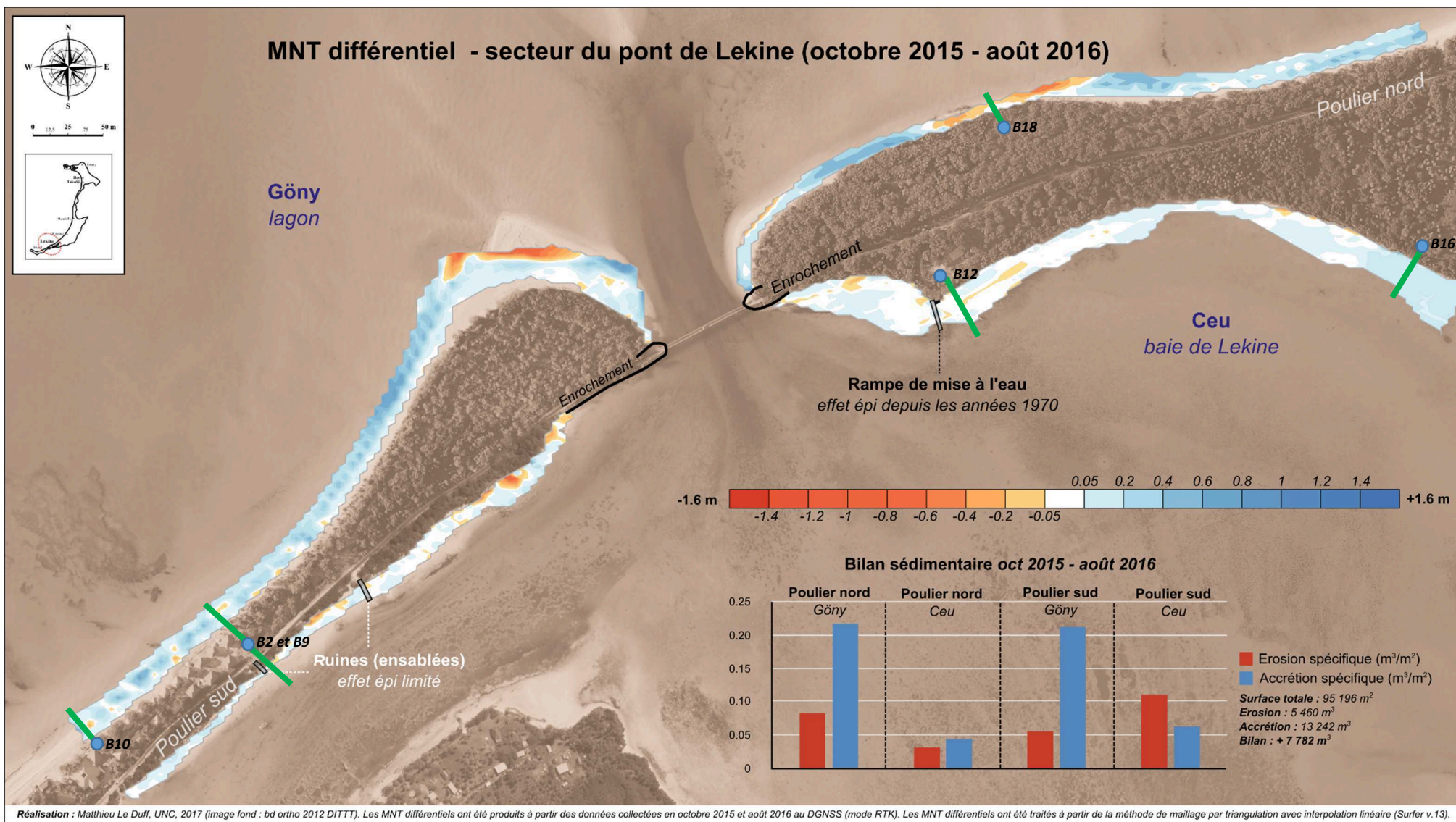
Figure 140 : MNT différentiel – Secteur du pont de Lekine (octobre 2015 – août 2016).
