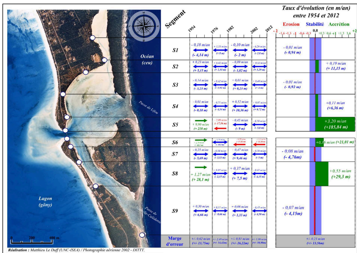
Figure 125 : Evolution de la position du trait de côte entre 1954 et 2012.
