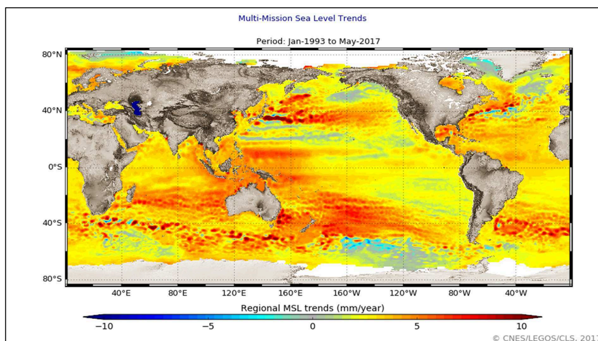
Figure 2: Carte globale de la distribution géographique des vitesses de variation du niveau de la mer (1993-2017) d'après Topex/Poseidon, Jason-1 et Jason-2. (Source : CNES-LEGOS-CLS).
