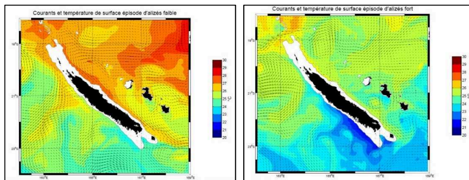
Figure 49 : schémas de la circulation durant l'absence et la présence d'événement d' upwelling en saison chaude. À gauche situation de vent alizé faible (31/12/2004), à droite situation de vent alizé fort et soutenu (9/11/2004). (Vega et al., 2005 ; Gardes et al., 2014)
