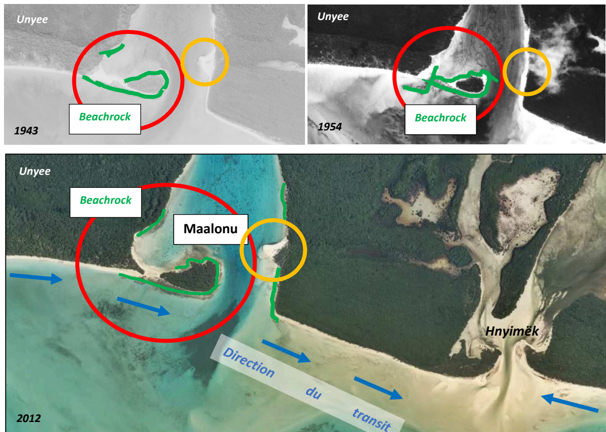
Figure 116 : Flèche en tombolo ayant pour base l'îlot Unyee et joignant l'îlot Maalonu. Source - Photographie : GIE Serail, 2012 ; DITTT, 1954 ; NARA, 1943.
