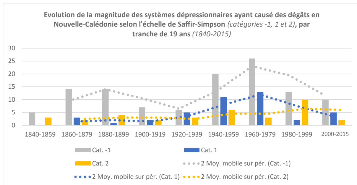
Figure 53 : Evolution de la magnitude des cyclones de catégorie 1 et 2, et systèmes dépressionnaires ayant causé des dégâts en Nouvelle-Calédonie, par tranche de 19 ans, sur la période 1840-2015.
