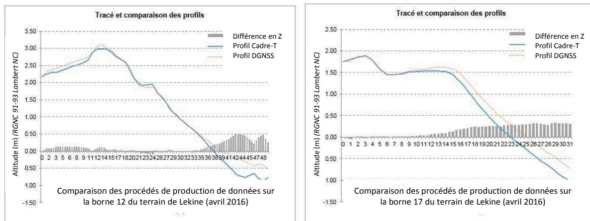
Figure 137 : Exemple de comparaison de profils levés au cadre-topomètre et DGNSS sur le site nord d'Ouvéa offrant un cumul d'erreur accentuant le décalage en bas de profils. Réalisation : Matthieu Le Duff, UNC, Profiler 3.1 (Cohen, 2014).
