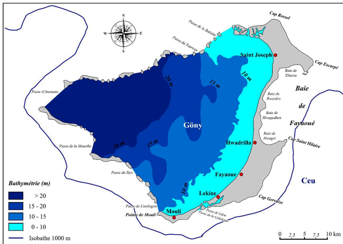
Figure 76 : Carte bathymétrique d'Ouvéa. (Source : SHOM).
