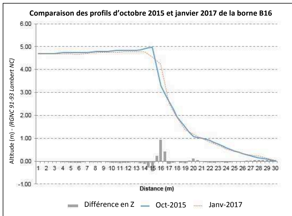
Figure 144 : Profils au cadre-topomètre de la borne 16 entre octobre 2015 et janvier 2017. (Réalisation : Matthieu Le Duff, UNC, Microsoft Excel, Profiler 3.2 (Cohen, 2014).
