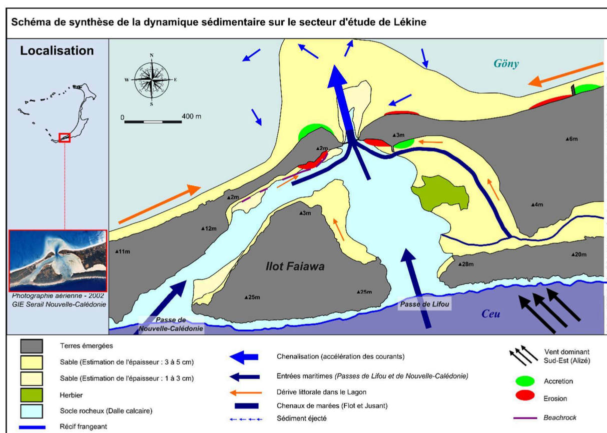
Figure 152 : Schéma de synthèse de la dynamique sédimentaire dans le secteur de la flèche en vis-à-vis du pont de Lekine.
