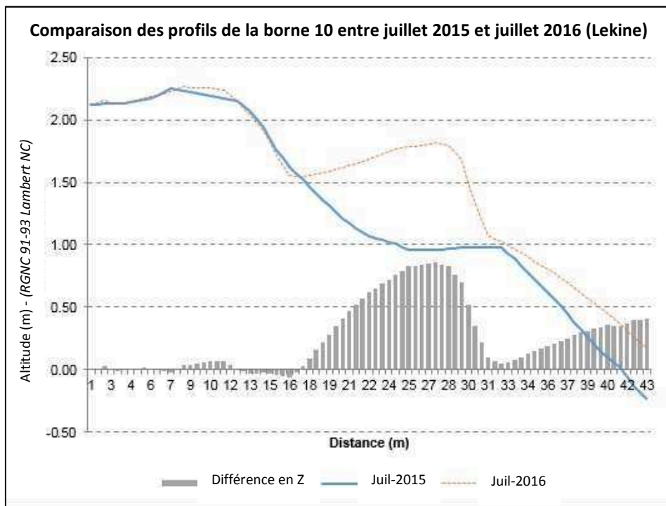
Figure 149 : Profils au cadre-topomètre de la borne 10 (Lekine) entre juillet 2015 et juillet 2016. (Réalisation : Matthieu Le Duff, UNC, Microsoft Excel, Profiler 3.2 (Cohen, 2014).
