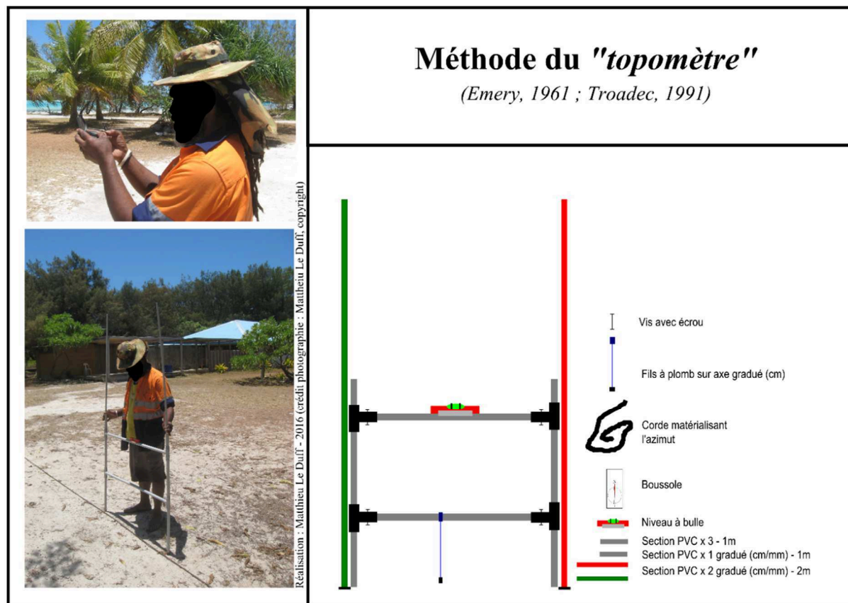
Figure 135 : Déclinaison de l'instrument « cadre-topomètre » de Troadec (1991).
