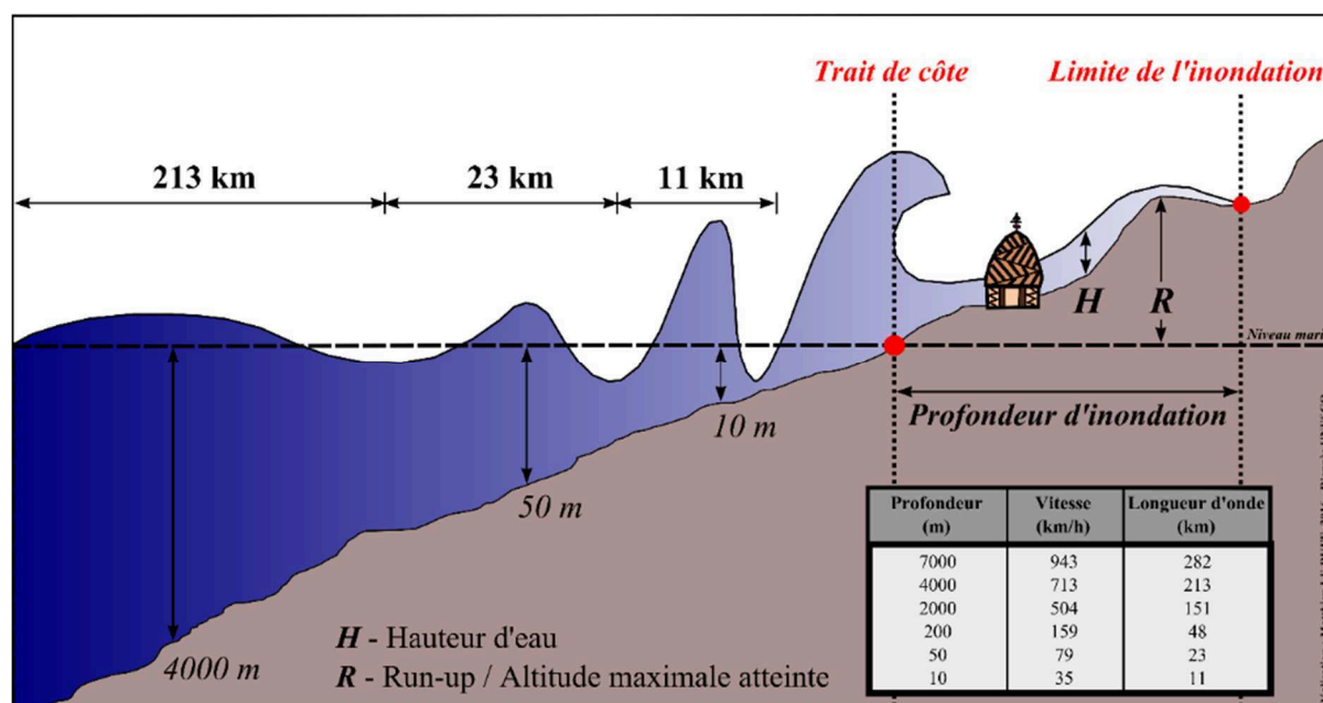
Figure 74 : Amplification / ralentissement des tsunamis à l'approche des côtes (shoaling effect) et éléments de caractérisation de la submersion marine associée aux tsunamis. (Source : Adapté de l'UNESCO).
