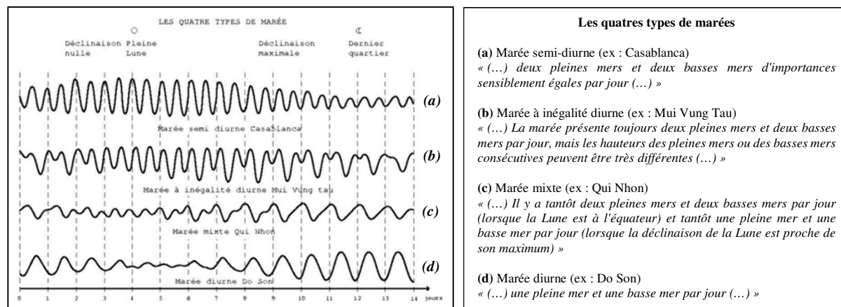
Figure 90 : Les différents types de marée (source : SHOM).
