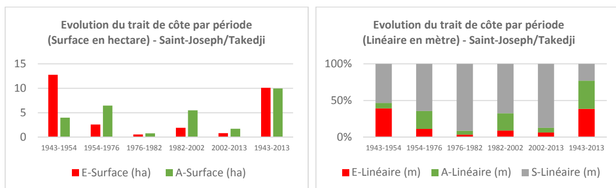
Figure 108 : Récapitulatif des évolutions observées sur le site d'étude de Saint-Joseph et Takedji, en surface (ha) et en distance linéaire (m). E : Erosion, A : Accrétion, S : non Significatif. Ces valeurs prennent en considération la marge d'erreur définie pour chaque période.
