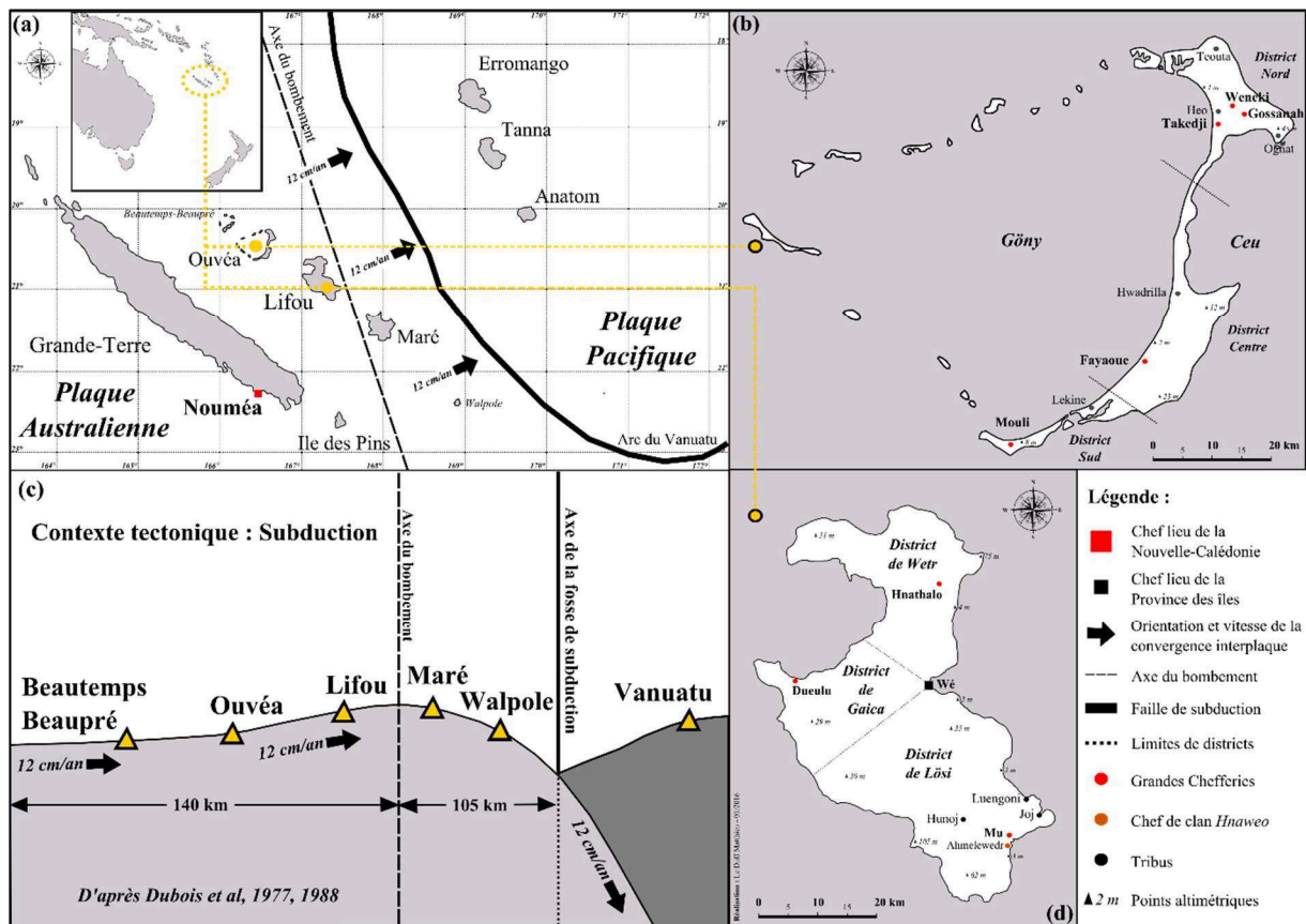
Figure 67 : Localisation des terrains d'études dans leur contexte tectonique régional.
