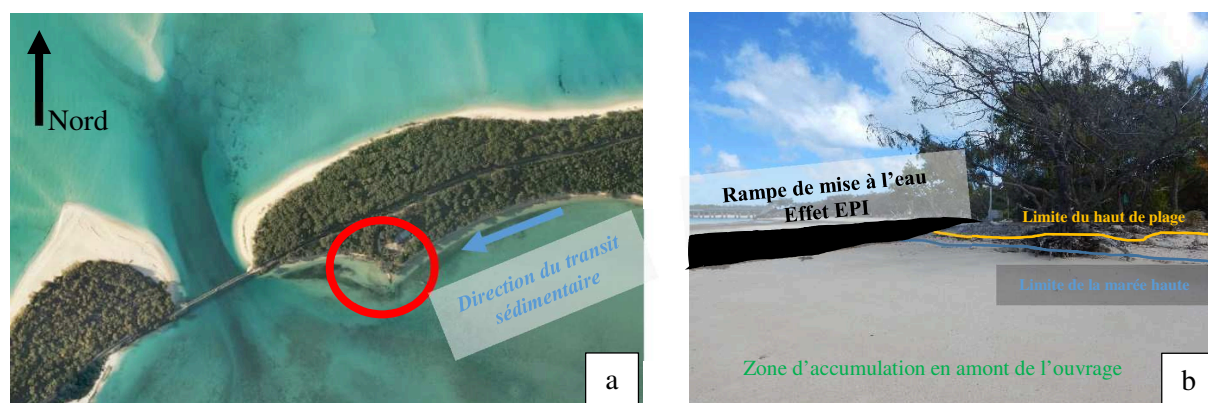
Figure 131 : Une plage qui disparaît quasi-entièrement à marée haute dans des secteurs bénéficiant d'ouvrages bloquant le transit sédimentaire. (a/ Image Satellite : GIE Sérail, 2012 ; b/ Photographie : Matthieu Le Duff).
