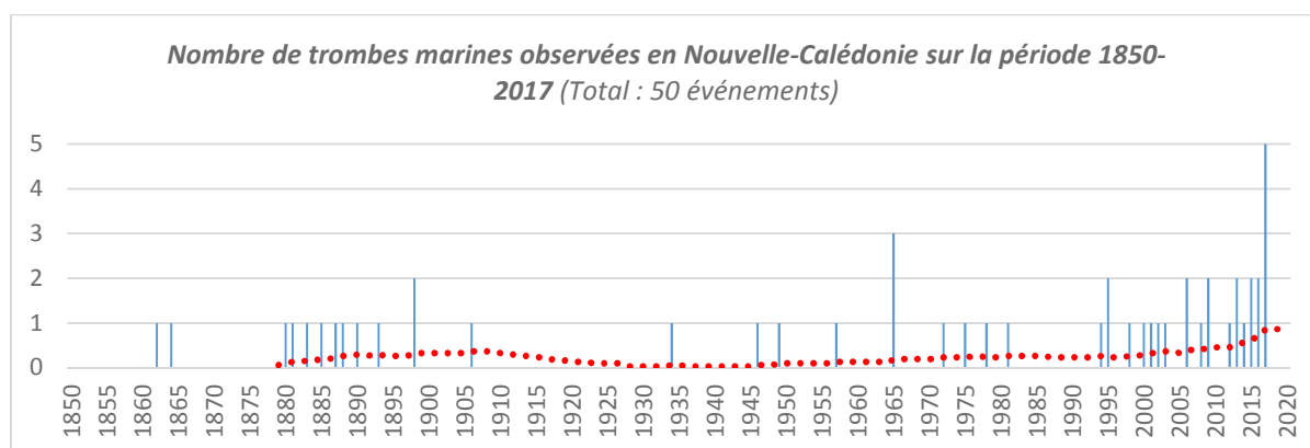
Figure 60 : Nombre de trombes marines observées en Nouvelle-Calédonie par an, sur la période 1850-2017 (total : 50 événements). Base de données construite à partir du dépouillement des archives et d'enquêtes de terrain. Courbe de tendance, moyenne mobile sur 30 ans, en rouge.
