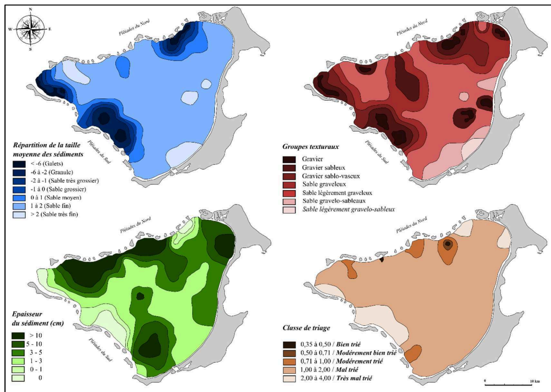
Figure 87 : Aperçu des conditions sédimentologiques du lagon d'Ouvéa, d'après Chevillon 1992. « Les indices statistiques des distributions de taille des grains (taille moyenne, triage, normalité et asymétrie) sont déterminés à partir des courbes semi-logarythmiques selon les formules de Folk & Ward (1957) et la classification de Wentworth (1922) » (Source : Chevillon, 1992).
