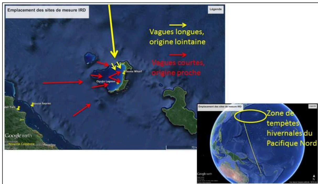
Figure 91 : Origine du régime des vagues captées dans le lagon d'Ouvéa, d'après Aucan (2015). Figure tirée du rapport OBLIC (2015) (pas de publication spécifique sur le sujet à ce jour à notre connaissance).
