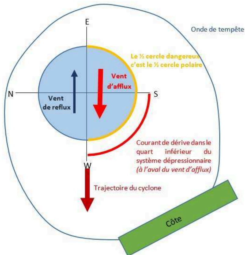
Figure 50 : Facteurs de formation de la marée tempête, la notion de 1/2 cercle dangereux et le vent d'afflux (inspiré de Mayençon, 1982).
