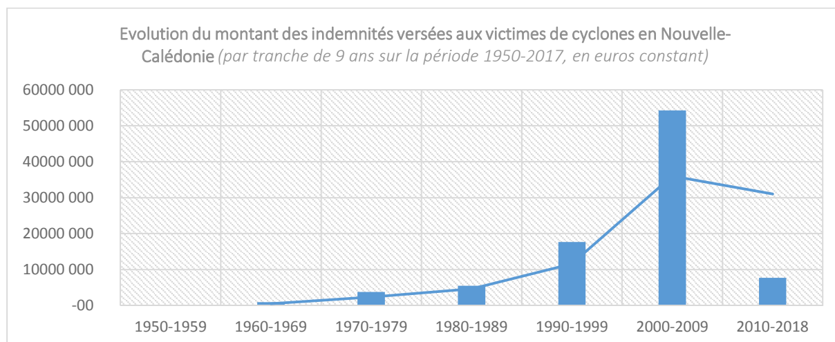
Figure 57 : Evolution du coût des impacts liée au passage des cyclones et systèmes dépressionnaires en Nouvelle-Calédonie, par tranche de 9 ans, sur la période 1950-2017, en euros constant.
