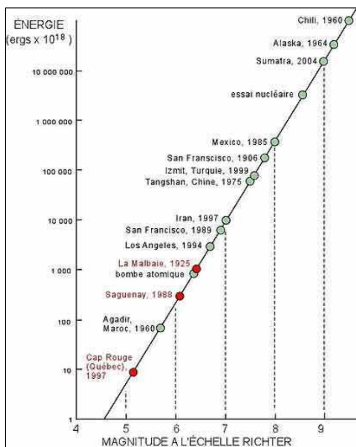
Figure 47 : Représentation classique de l'échelle de Richter (source : Internet).
